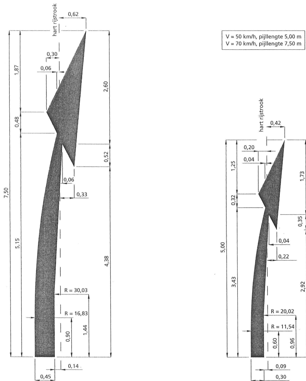
Figuur 2.19. Verdrijfpil voor bubeko en bibeko
